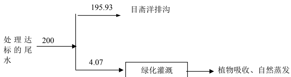
图 2-2 建设项目营运期水平衡图 (m³/d)
